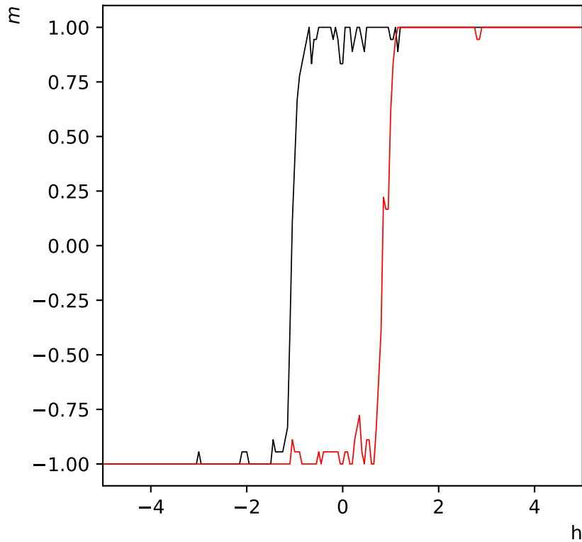
Hystérésis de l'aimantation réseau de taille L=6 - h=5 à T=2.0
