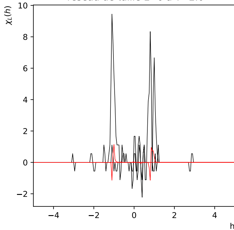
\chi_L(h) réseau de taille L=6 à T=2.0
